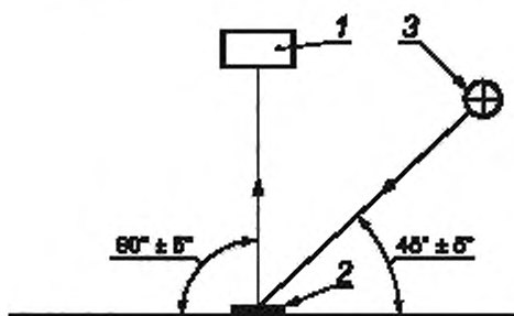
1 — спектрофотометр или колориметр для измерения координат цветности, спектрофотометр, колориметр или яркомер для измерения коэффициента яркости; 2 — дорожная разметка; 3 — источник света
