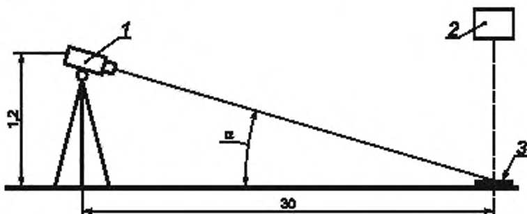
1 — фотоприемник; 2 — источник света типа D65 по ГОСТ 7721; 3 — поверхность разметки, размеры в метрах
