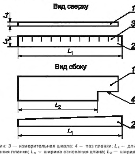
Рисунок 1 — Схема высотомера для определения высоты выступающей горизонтальной дорожной разметки над поверхностью, на которую она нанесена
