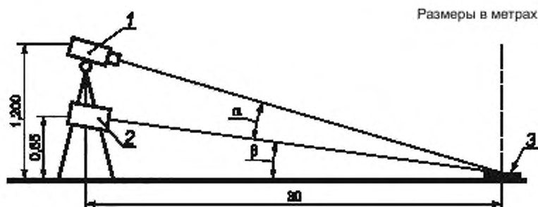
Рисунок 2 — Условия определения коэффициента световозвращения горизонтальной дорожной разметки
